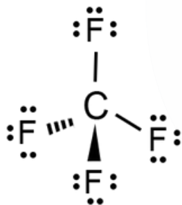
CF 4
