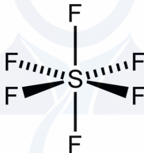
SF 6
